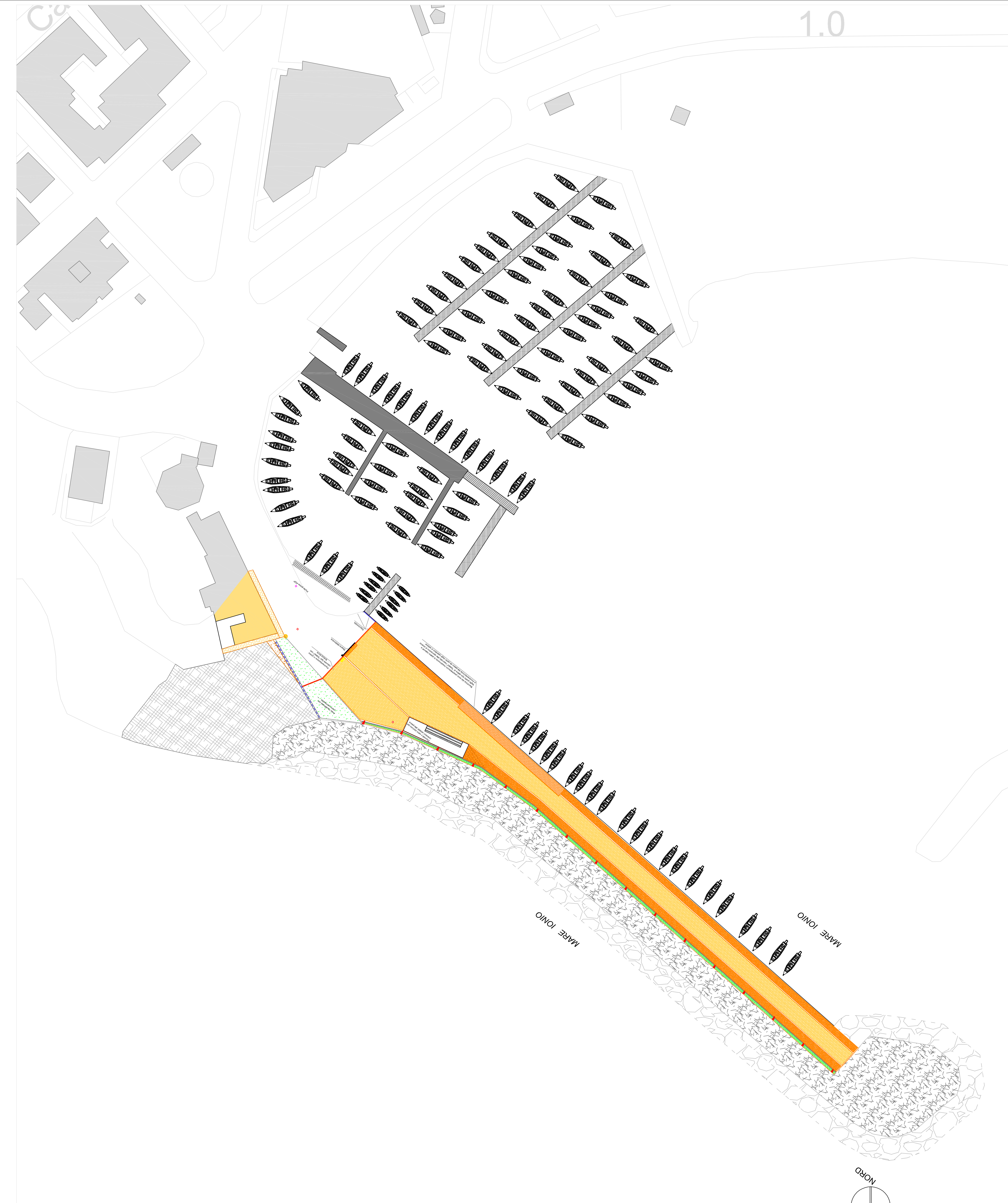
Planimetria del Porto di San Giovanni - Scala 1:500
