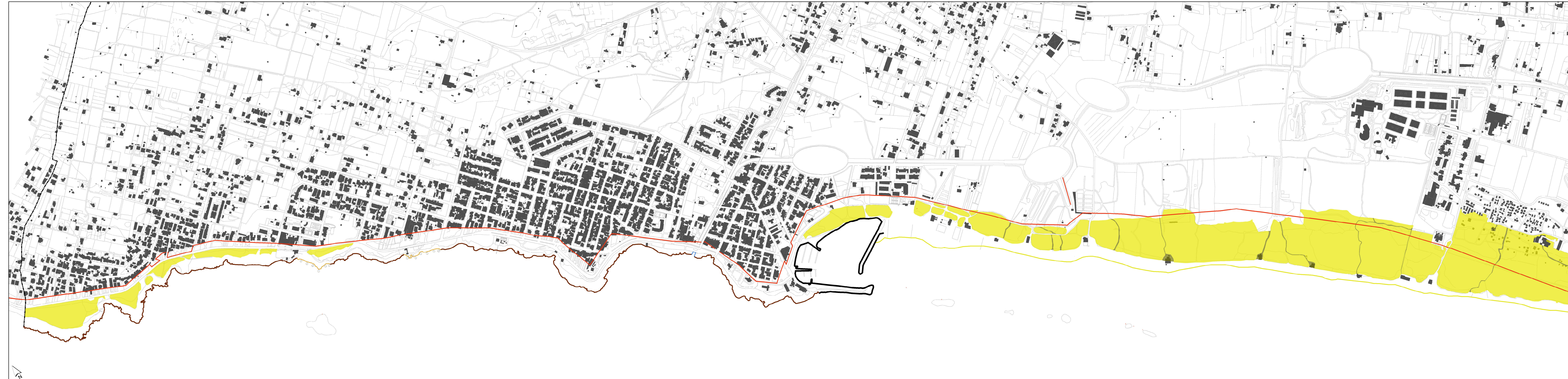
TAV. A 4 MORFOLITOLOGIA COSTIERA E CARATTERIZZAZIONE DELLA COSTA
